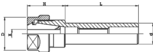
Pince DIN 6499B
